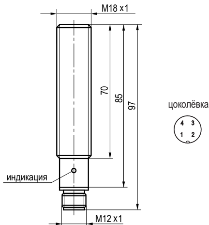
Габаритный чертёж
